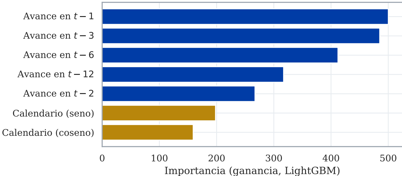
Importancia de características para el avance mensual (FAD)
