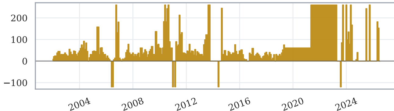
(b) Primera diferencia: estacionaria y extrapolable
