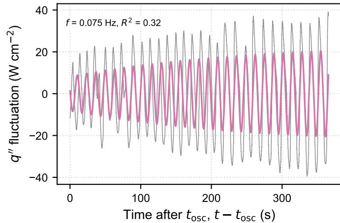
(d) P_{\text{load}} = 250 \text{ W}
