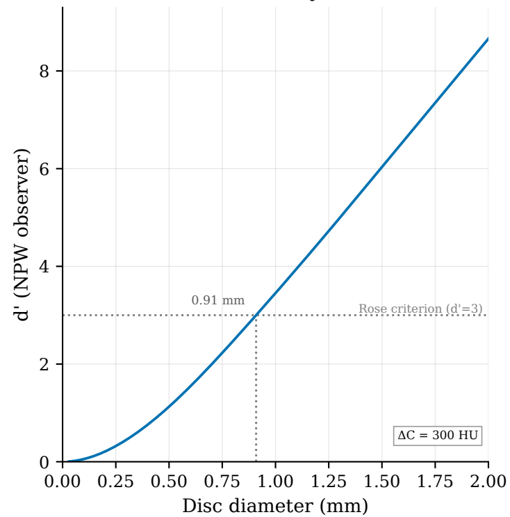
Detectability ( d' )
