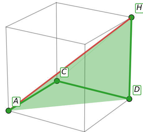
(d) T_3 = [A, C, D, H] , \text{vol}(T_3) = -\frac{1}{6}
