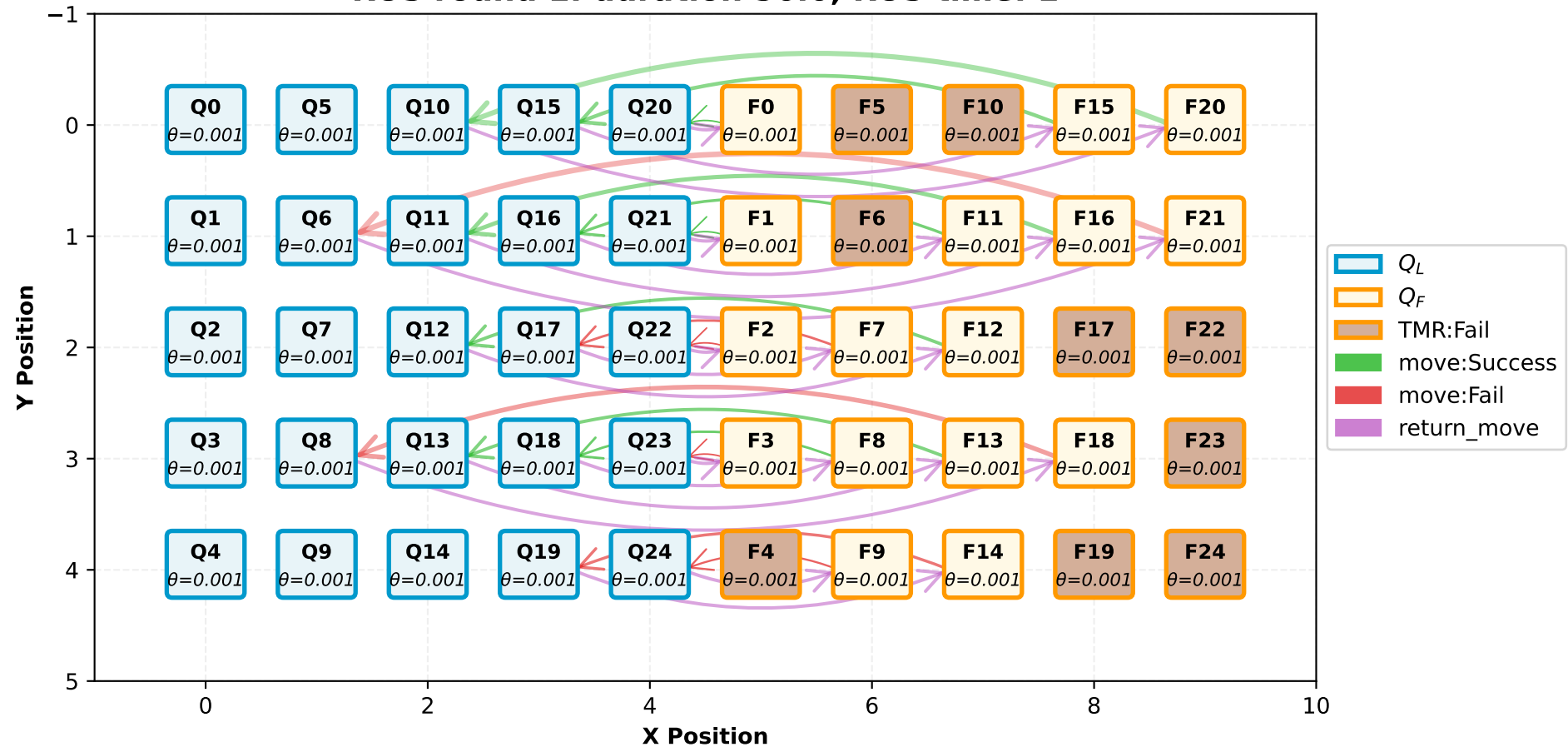
RUS round 1: duration 56.0, RUS time: 1
