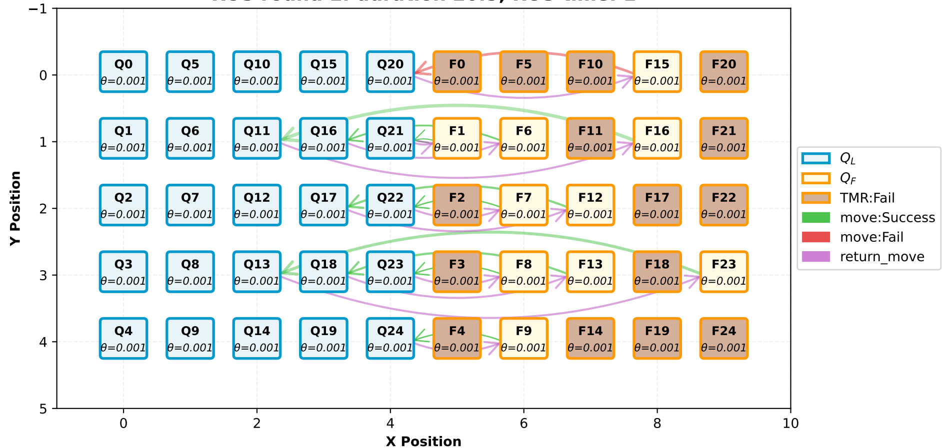
RUS round 1: duration 20.5, RUS time: 1
