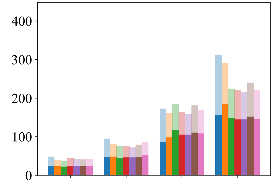
X layer
