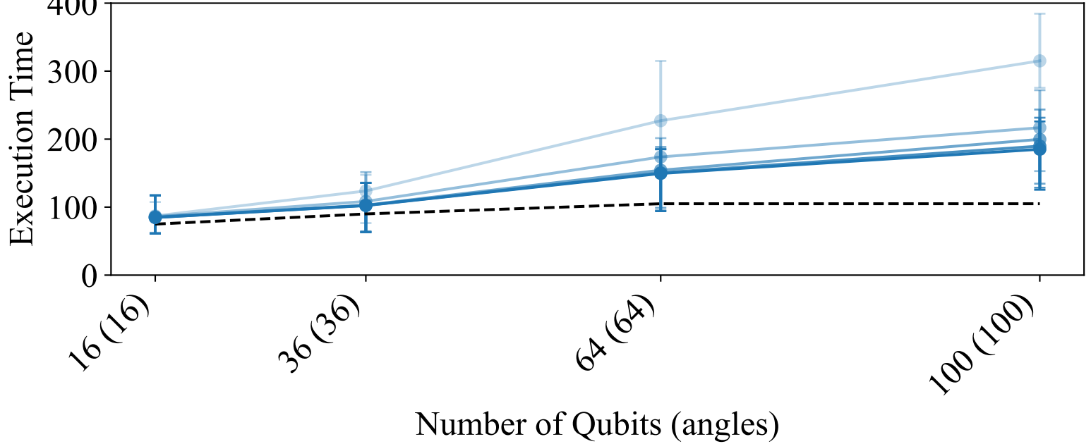
X layer
