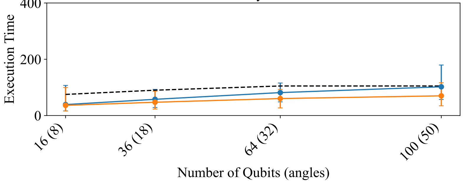
X layer
