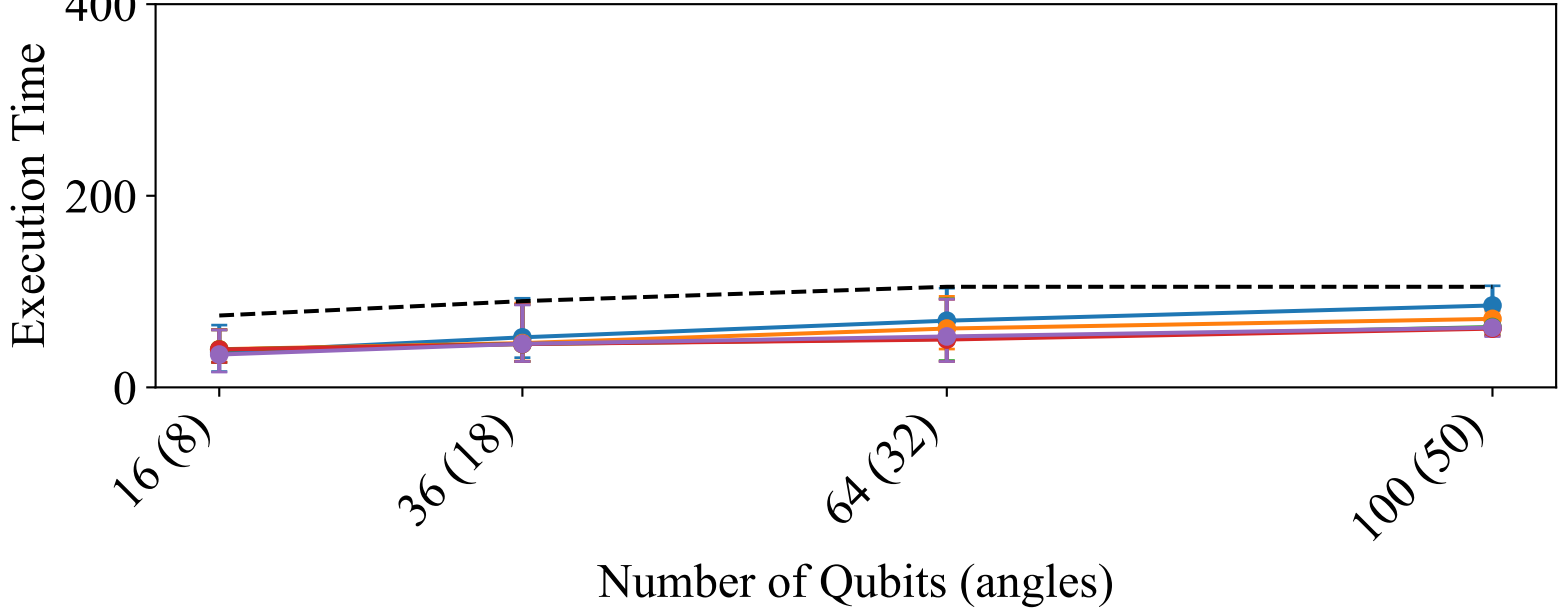
X layer
