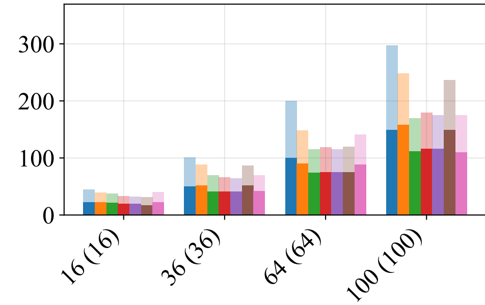
X layer
