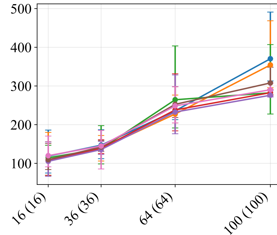
X layer
