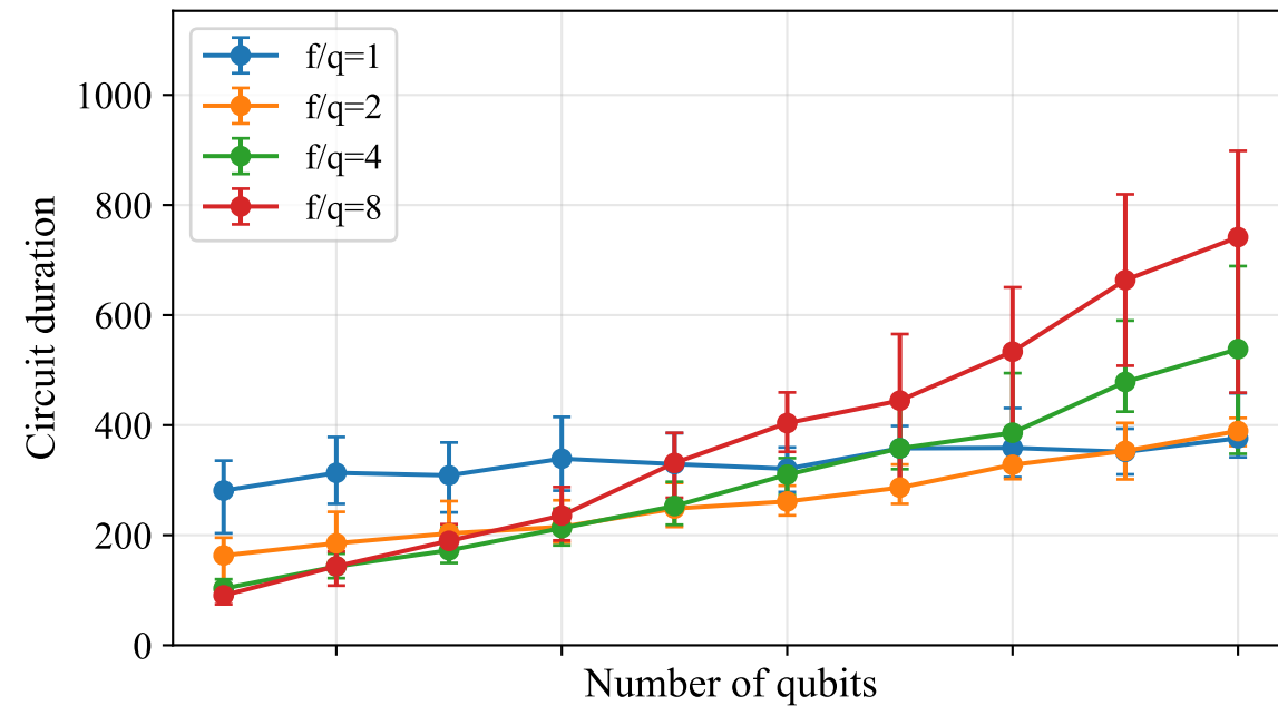
distance-7, LER: 1e-08
