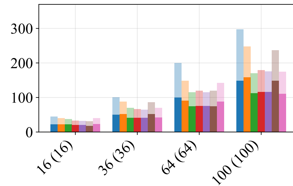
X layer
