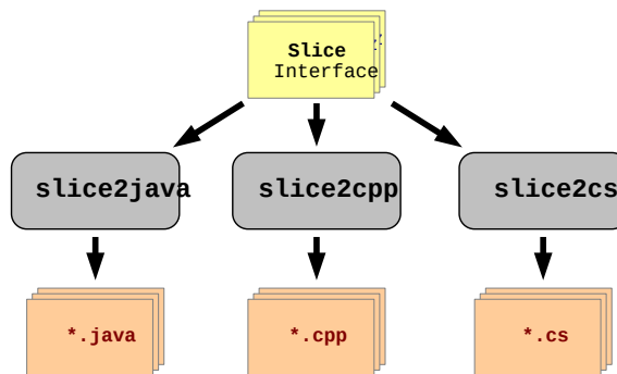
FIGURA 1.3: ICE genera un compilador de interfaces para cada lenguaje soportado
