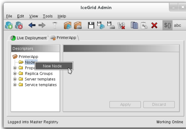
FIGURA 3.8: IceGrid Admin: Creación de un nodo
