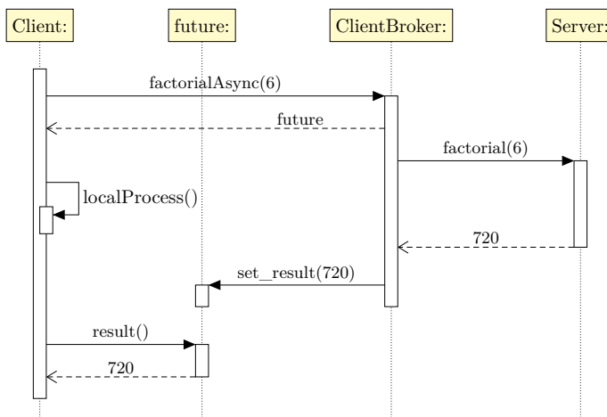
FIGURA 5.1: Invocación asíncrona (el cliente recoge el resultado más tarde)
