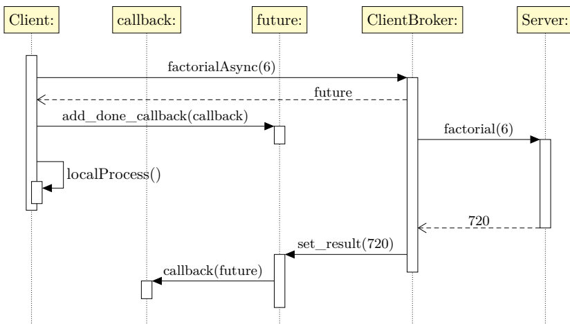
FIGURA 5.2: Invocación asíncrona (objeto callback )
