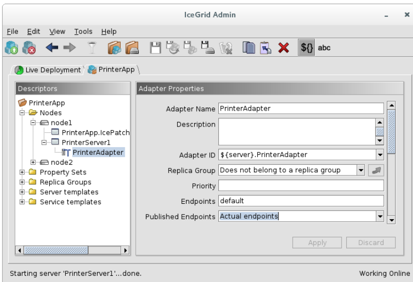
FIGURA 3.11: IceGrid Admin: Configuración del adaptador de objetos
