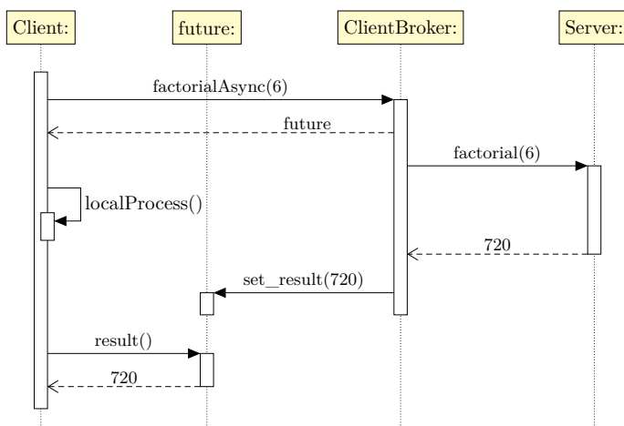
FIGURA 5P.1: Invocación asíncrona (el cliente recoge el resultado más tarde)
