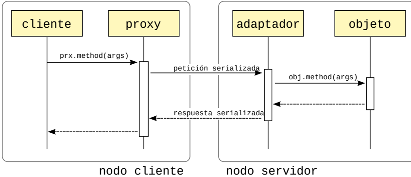
FIGURA 1P.2: Diagrama de secuencia de una invocación remota síncrona
