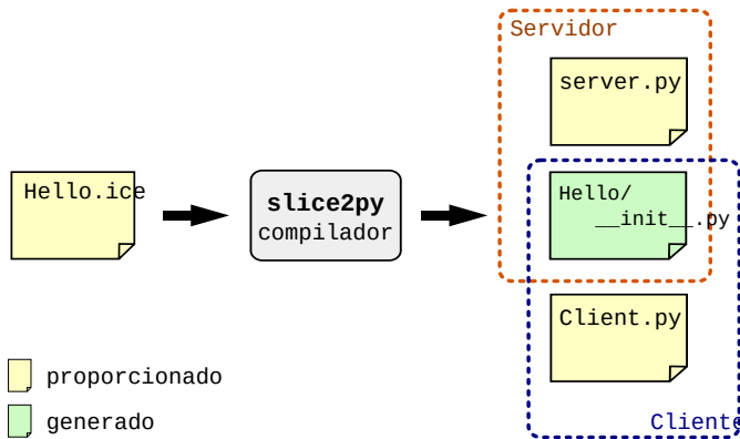
FIGURA 1P.4: Esquema de compilación de cliente y servidor en Python
