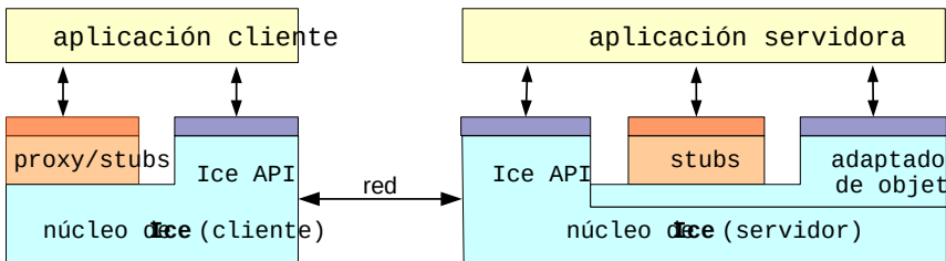
FIGURA 1P.1: Componentes de una aplicación ICE
