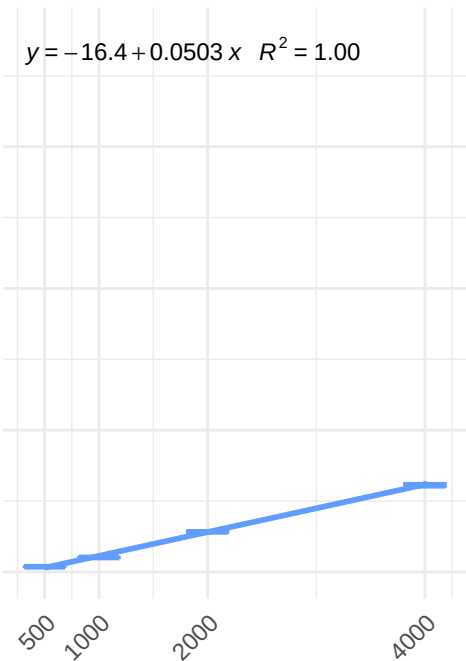
benchmarkJoinPSM
