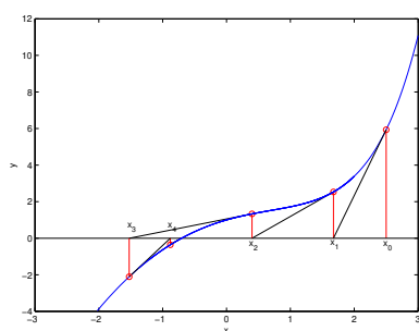
(e) iteración 4
