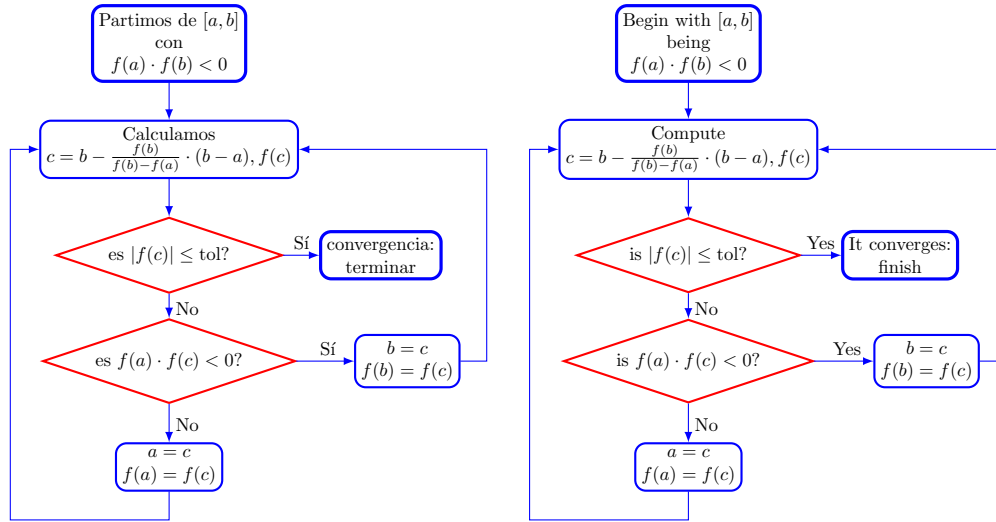
Figura 6.6: Diagrama de flujo del método de interpolación lineal
