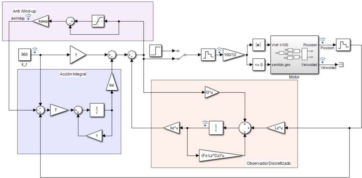
Figura 5.15: Sistema completo para alimentar el motor real, empleando el esquema de Simulink (fig. 4.1) para manejar el motor real. Los bloques añadidos antes del motor permiten pasar de tensión en voltios a señal de PWM
