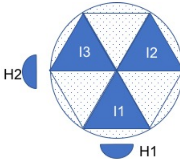
Figura 1.7: Esquema de la posición relativa de los sensores de efecto Hall (H1 y H2) y los imanes permanentes para el encoder del motor EMG30. En la posición que se muestra, H2 estaría en un flanco de subida o bajada –según la dirección de giro del motor– y H1 estaría en el centro de un pulso
