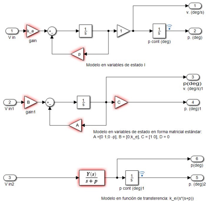
Figura 5.1: Esquemas de Simulink para el modelo del motor ideal
