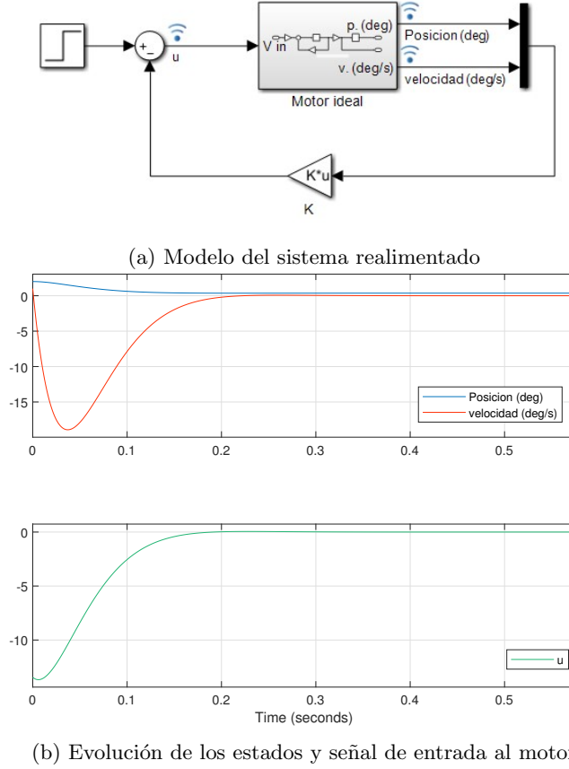
Figura 5.9: Realimentación de estados para el motor ideal
