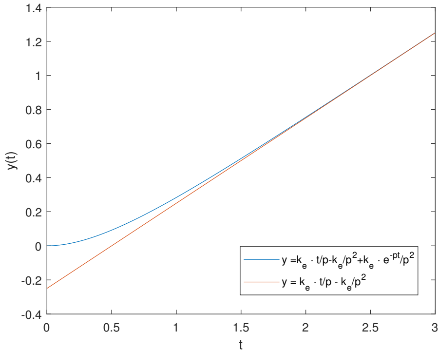
Figura 4.3: Respuesta de un motor de cc a un voltaje de entrada escalón
