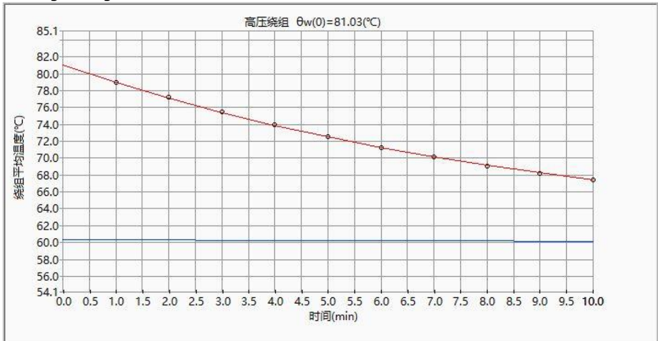
F1 HV winding temperature curve
