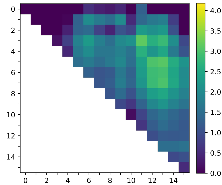
olmo-1b-sft
