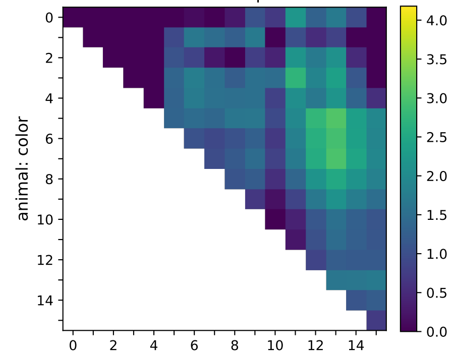
olmo-1b-dpo
