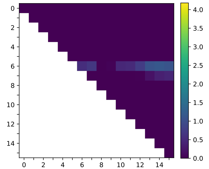
olmo-1b
