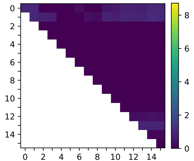
olmo-1b
