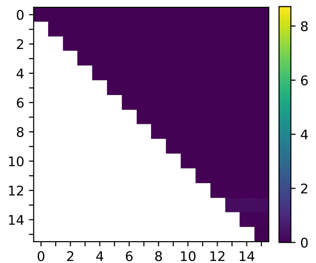
olmo-1b-dpo
