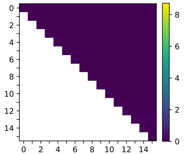
snarks
