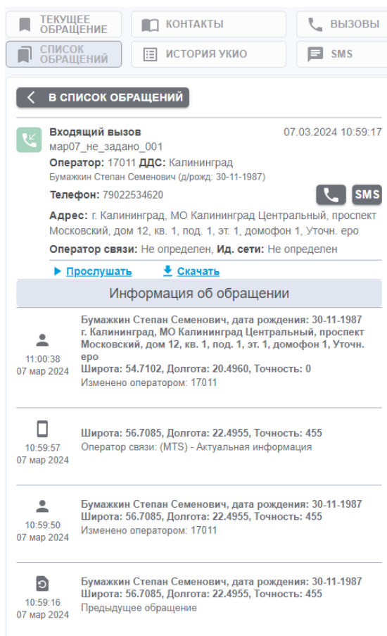
Рисунок – Вкладка СПИСОК ОБРАЩЕНИЙ – Режим отображения деталей обращения
