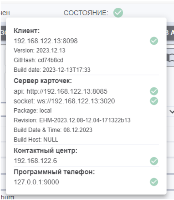
Рисунок – Индикатор состояния рабочего места
