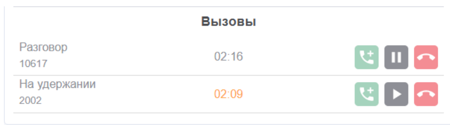
Рисунок – Вкладка Вызовы – Список вызовов
