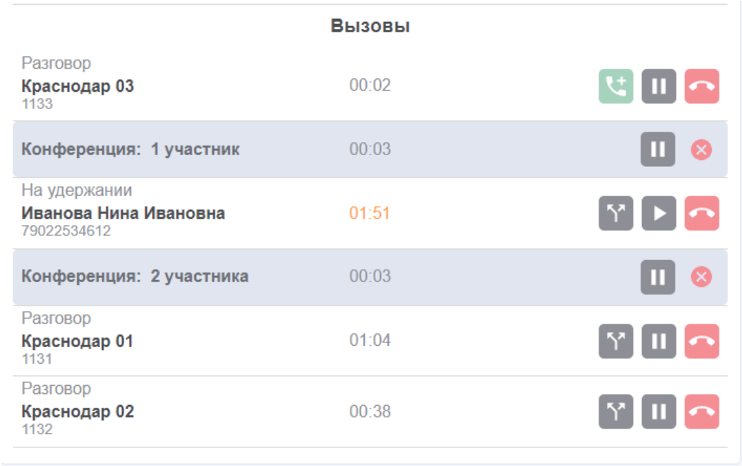
Рисунок – Список конференций
