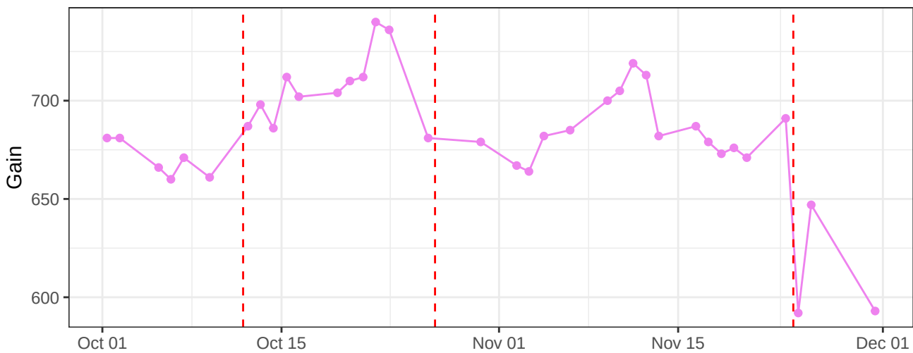
V16-A_Gain
