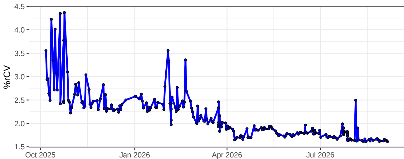
B14-% rCV
