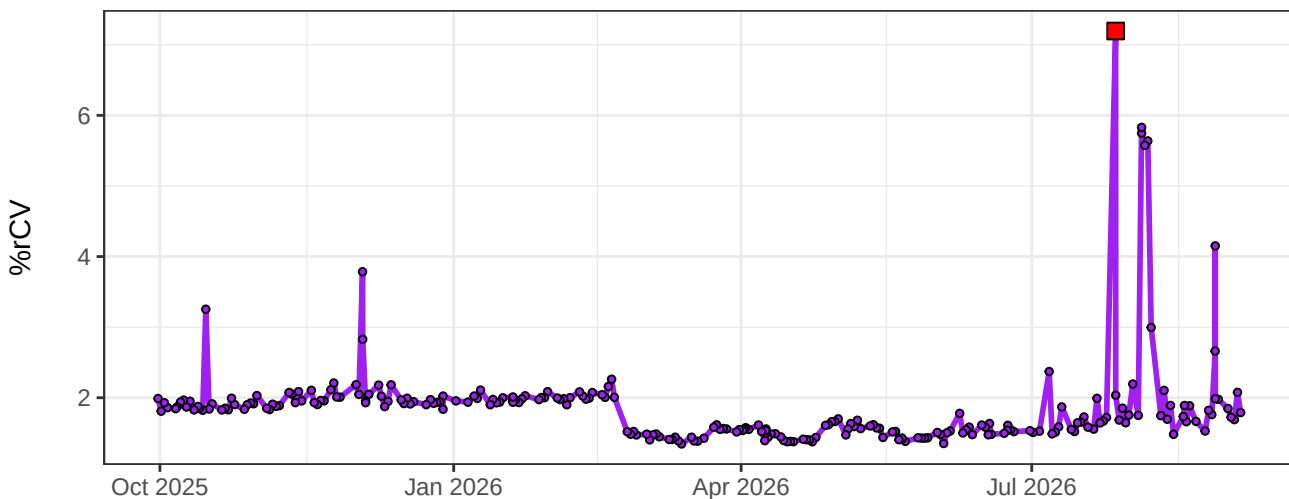
UV15-% rCV
