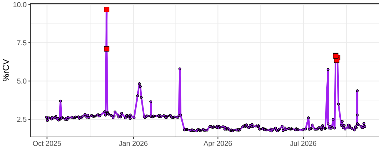
UV16-% rCV
