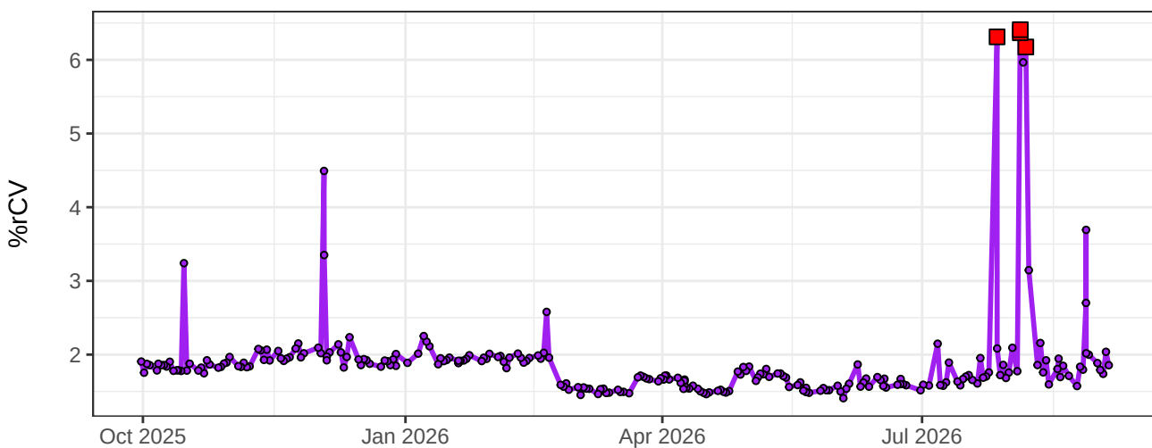
UV16-% rCV
