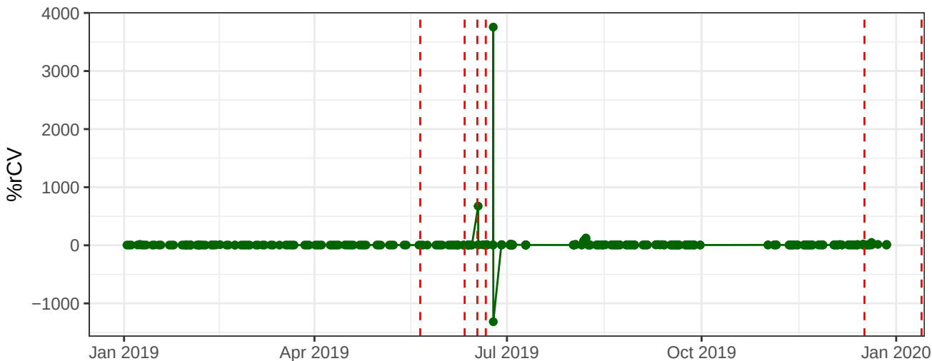
Y615-A-% rCV
