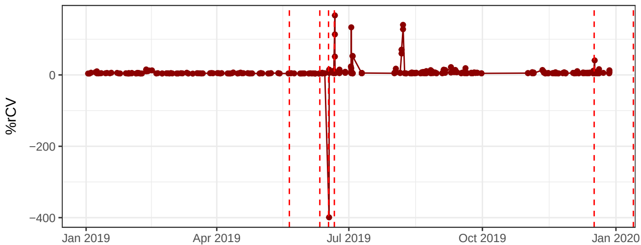
R730-A-% rCV
