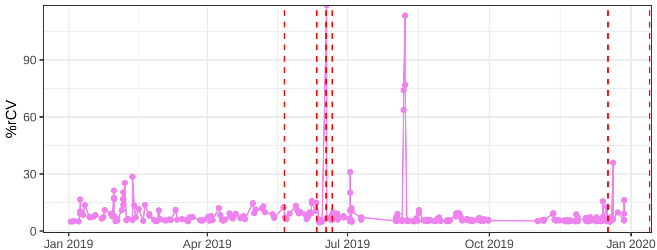
B530-A-% rCV
