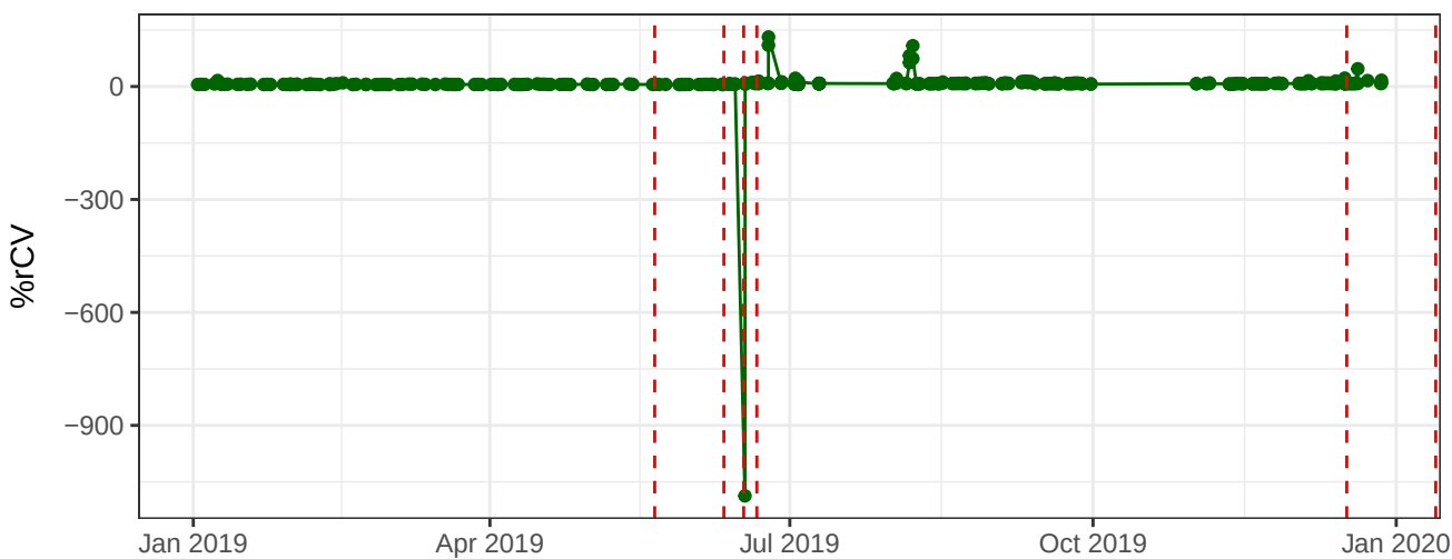
Y710-A-% rCV
