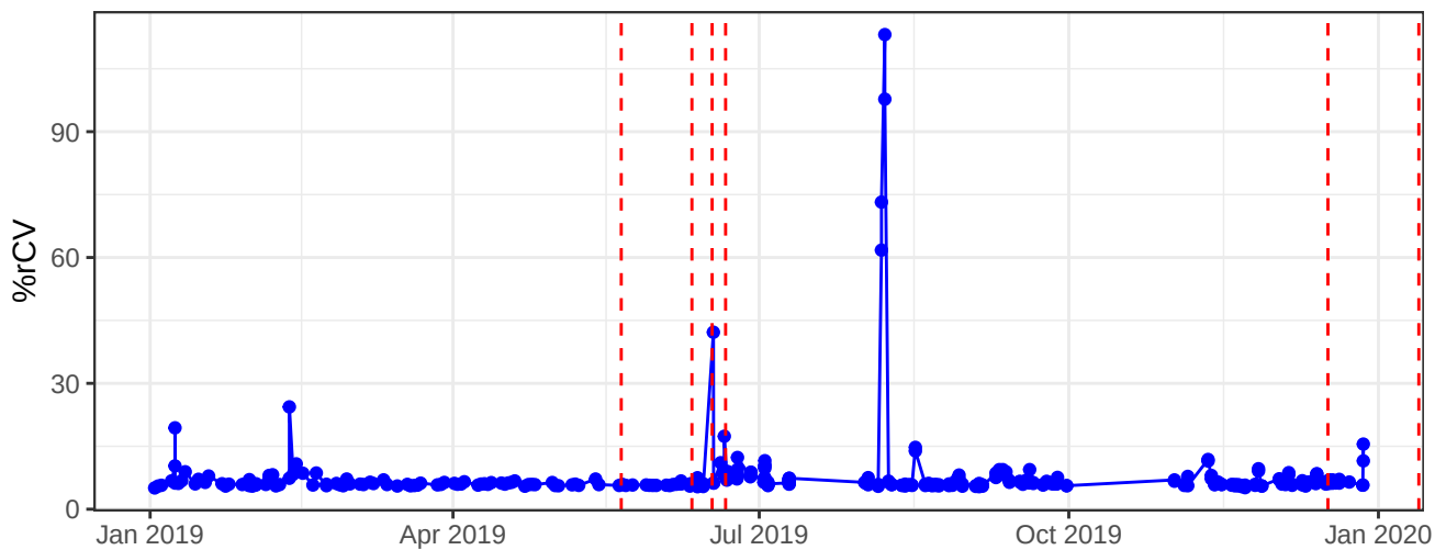
B710-A-% rCV
