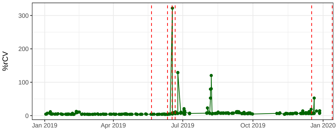
Y710-A-% rCV
