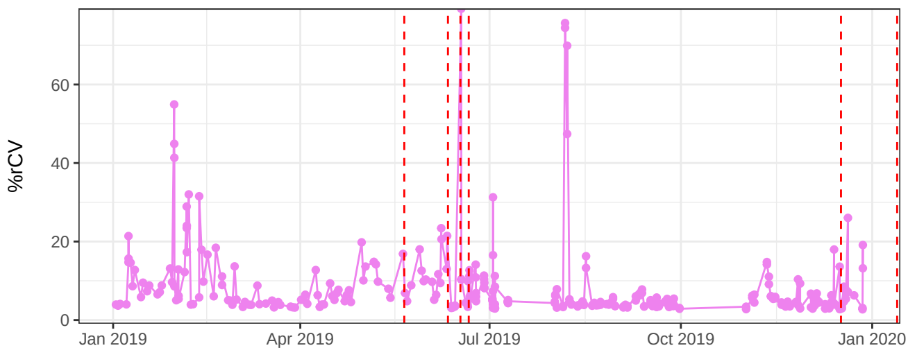
V610-A-% rCV
