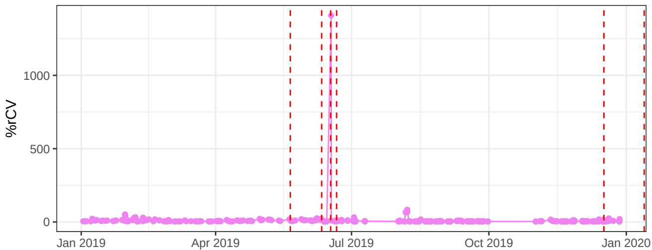
V525-A-% rCV
