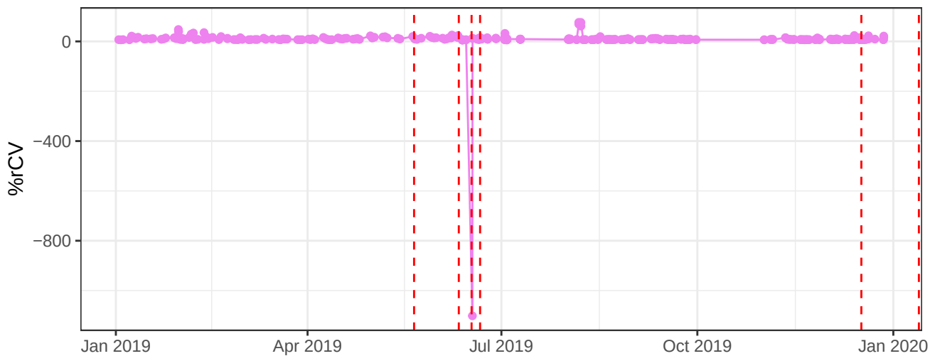
V610-A-% rCV
