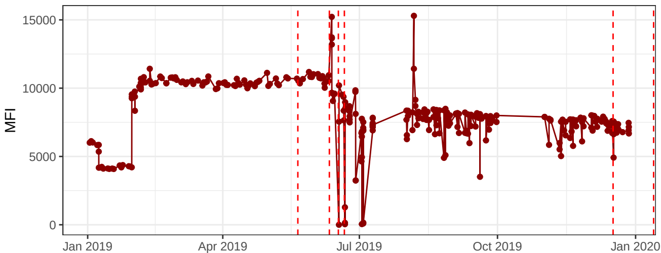
R730-A
