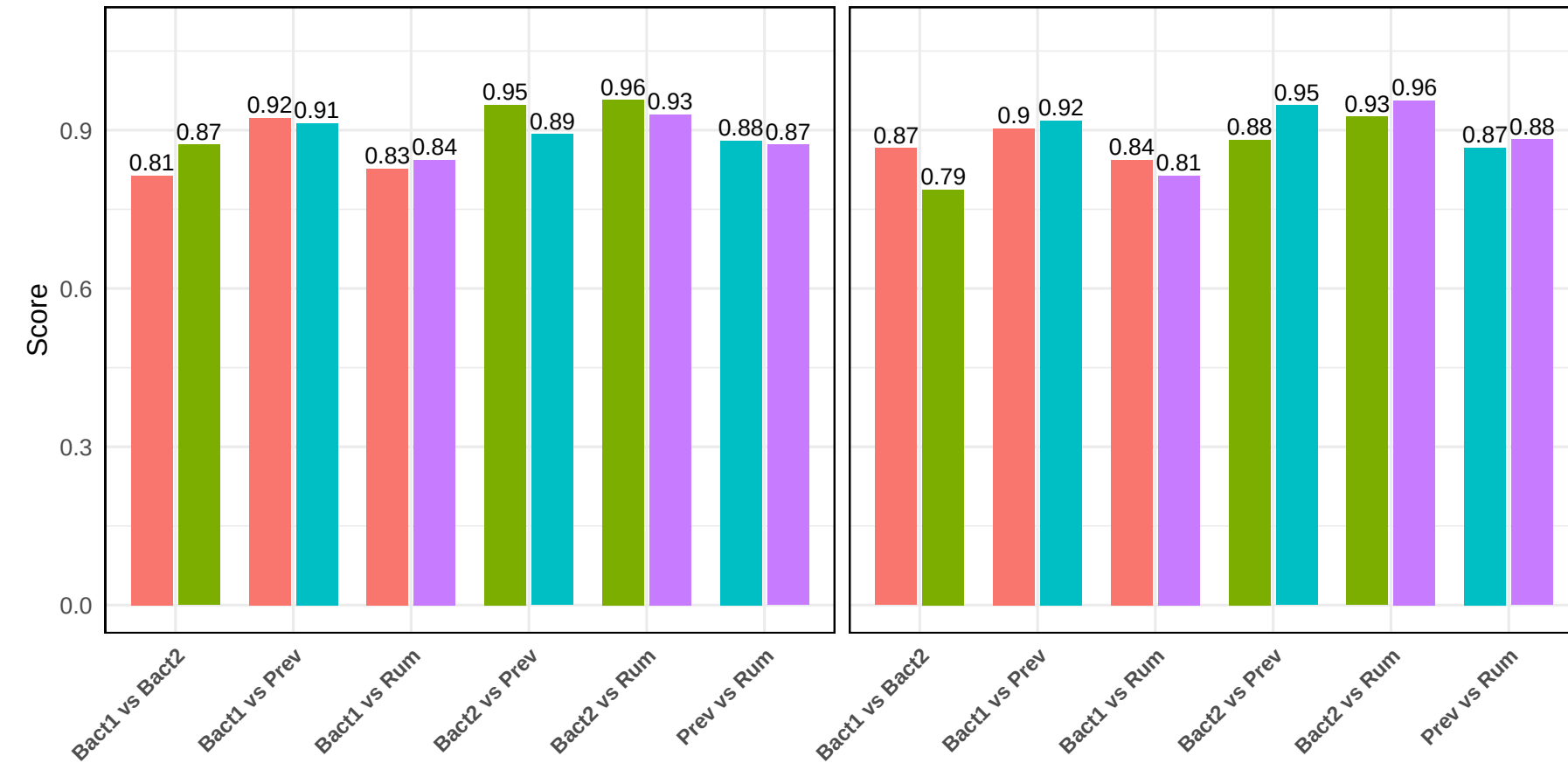
SVM
