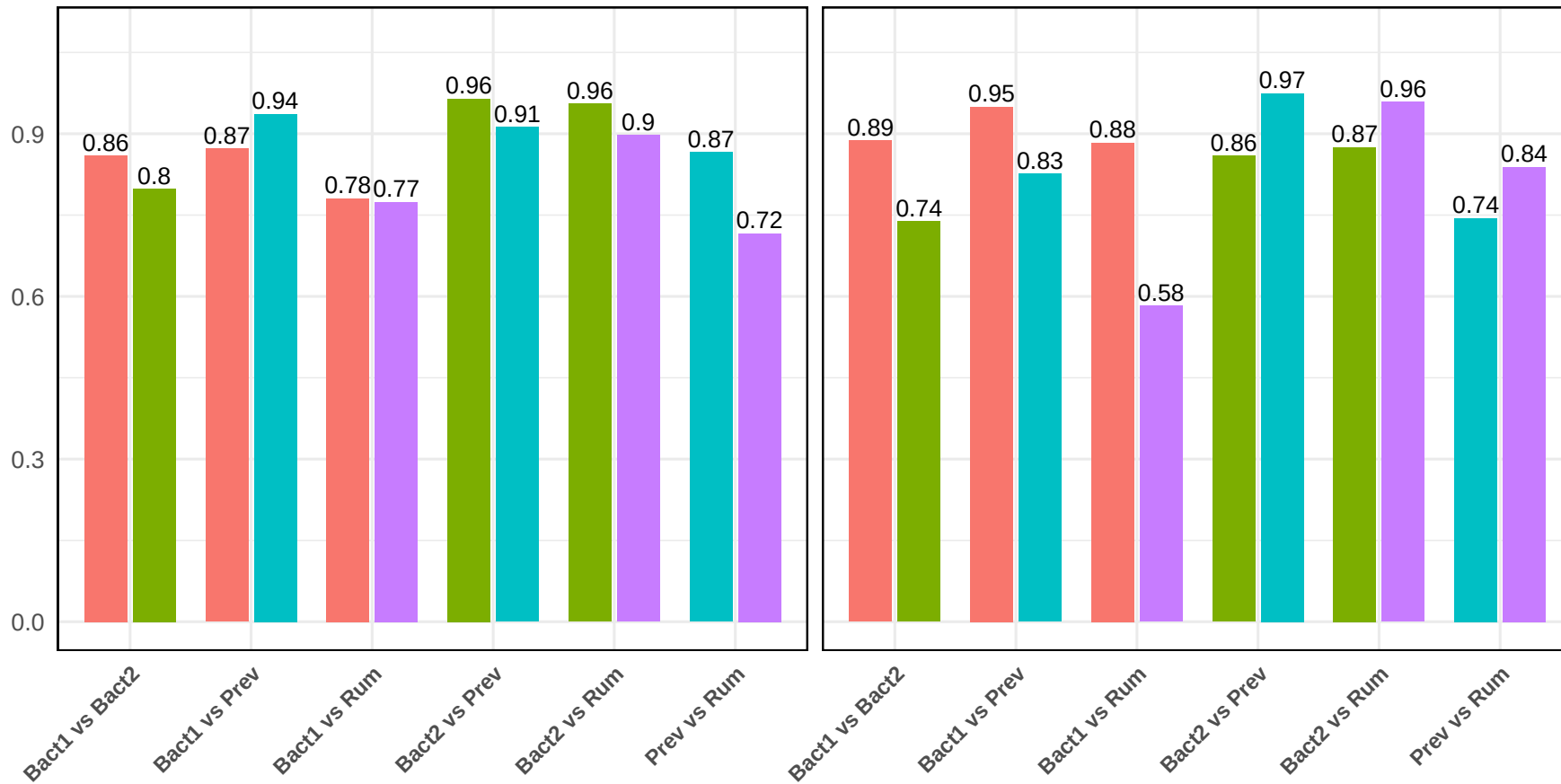
SVM
