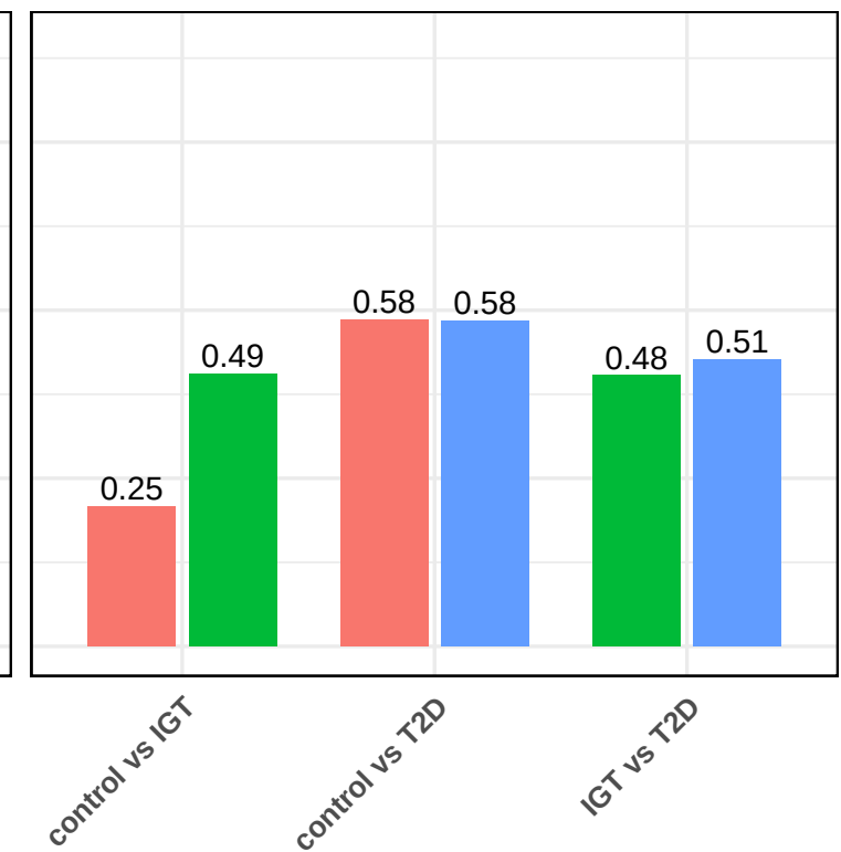
Precision
