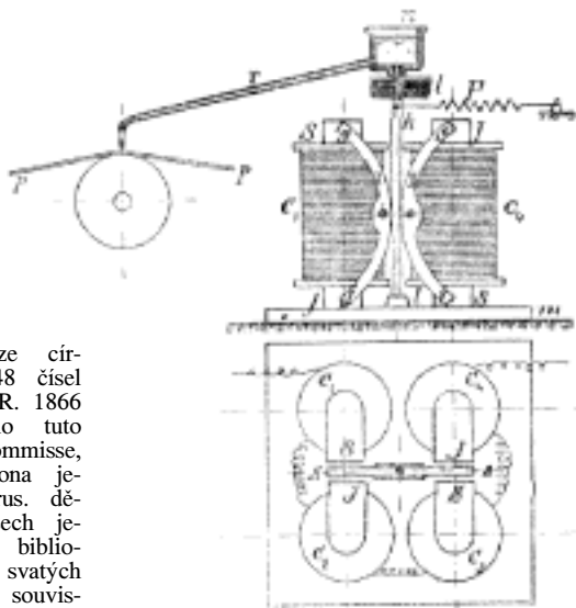
Č. 4490. Undulátor Lauritzenův.
