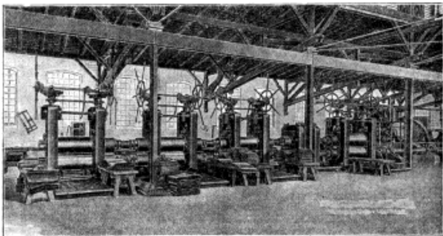
Č. 4529. Pohled do válcovny na válcování olova.
