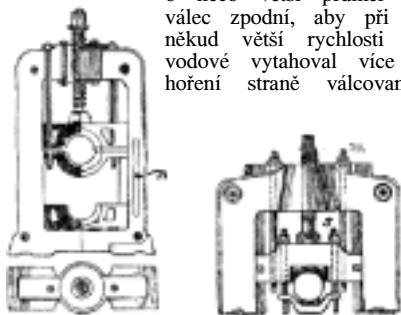
Č. 4520. Stojan složení dvouválcového. Č. 4521. Uložení válců podle Daelena.
