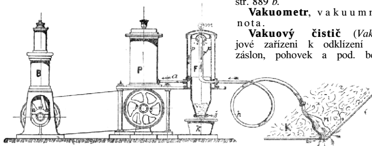
Č. 4513. Vakuový čistič.
