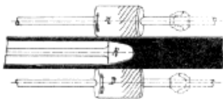
Č. 4527. Válcování rour dle způsobu Mannesmannova.
