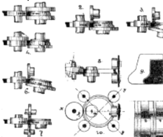
Č. 4525. Válcování nákolků.
