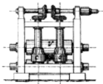
Č. 4517. Válcové složení univerzální.
