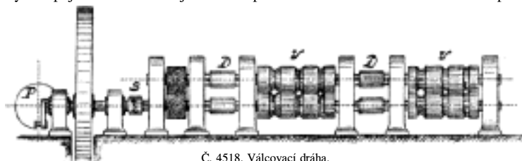
Č. 4518. Válcovací dráha.
