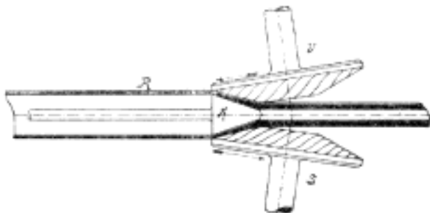
Č. 4528. Vtahování kusu mezi válce při válcování dle Mannesmann.
