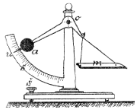
Č. 4512. Váhy poštovní.
