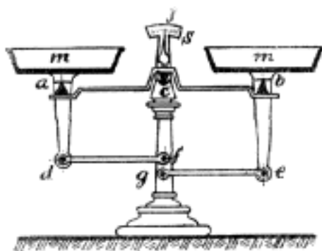
Č. 4509. Robervalovy váhy.
