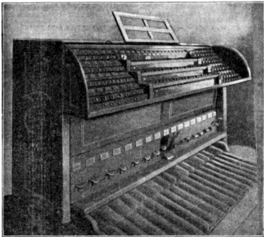
Č. 4537. Hrací stolec Petrových varhan v Karlině.
