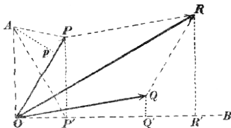
Č. 4540. Varignonova věta.
