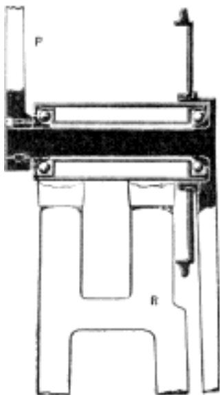
Č. 4559. Uložení hřídele klikového.
