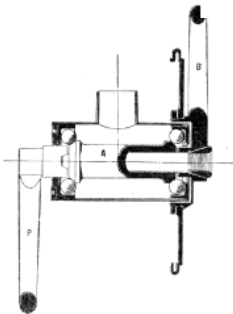
Č. 4560. Uložení hřídele klikového.
