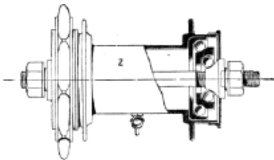
Č. 4561. Uložení hřídele zadního.
