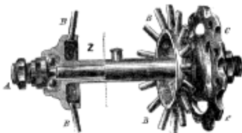
Č. 4558. Uložení zadního kola, paprsky radiálně zapuštěné.
