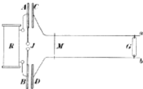
Č. 4632. Stojaté vlny elektrické v drátech.
