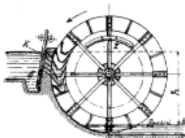
Č. 4639. Vodní kolo se zadním dopadem.
