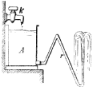
Č. 4647. Vodotrysk periodický.
