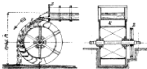
Č. 4638. Vodní kolo na svrchní vodu.
