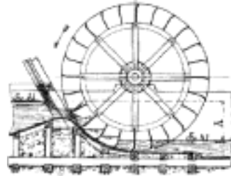
Č. 4641. Kolo Züppingerovo.
