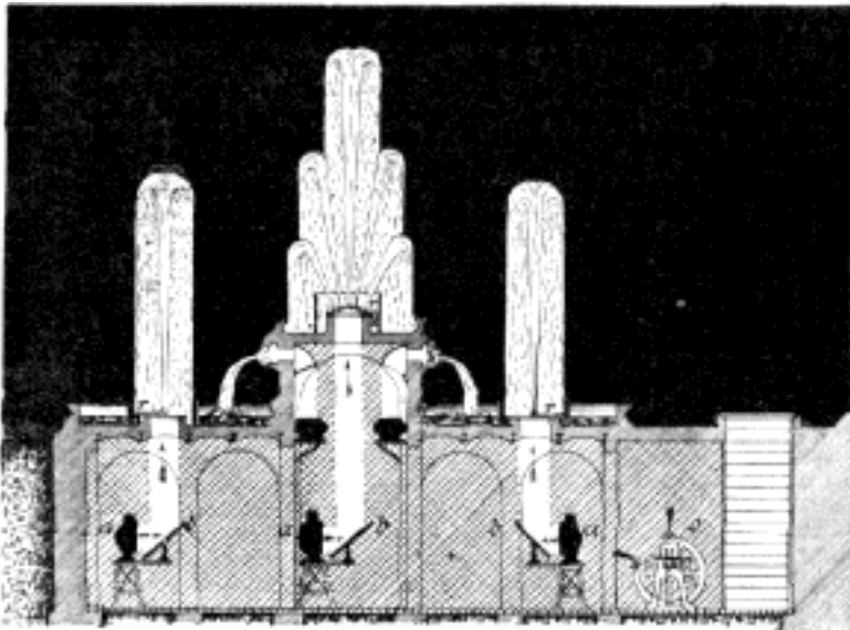
Č. 4648. Vodotrysk světelný.
