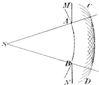
Č. 4631. Princip Huygensův.
