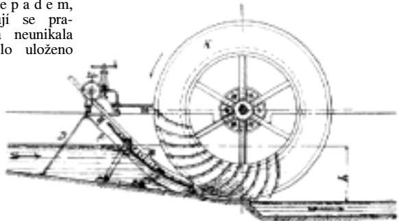
Č. 4642. Kolo Poncelotovo.
