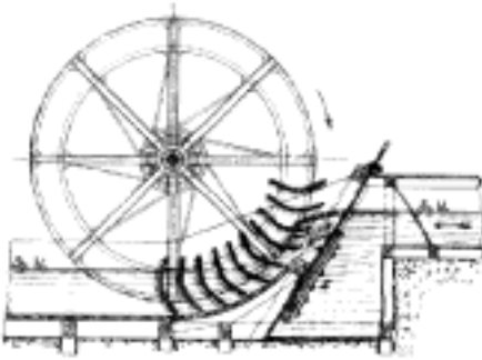
Č. 4640. Vodní kolo s přepadem.
