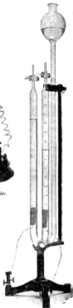
Č. 4653. Voltametr Hoffmannův.
