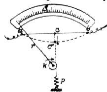
Č. 4660. Voltmetr kalorický.
