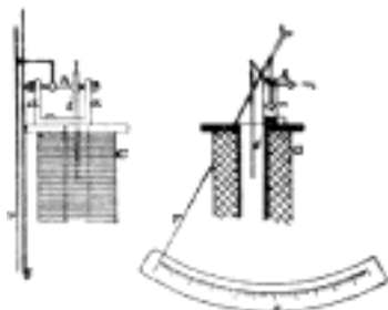
Č. 4657. Voltmetr AEG.
