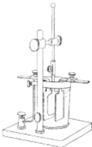
Č. 4654. Voltametr na měď.
