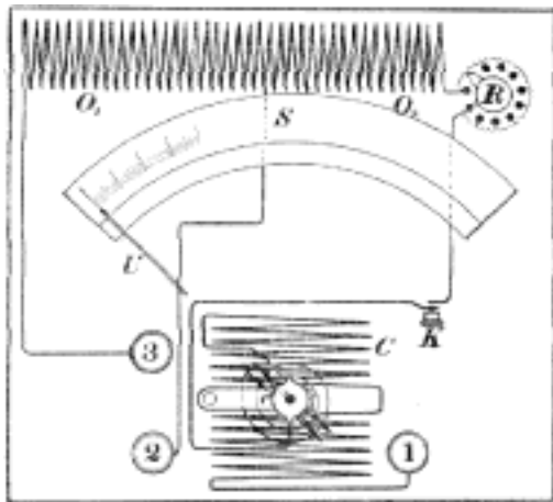
Č. 4656. Voltmetr Westonův.
