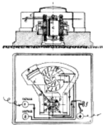
Č. 4659. Voltmetr Westonův.
