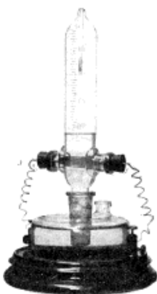
Č. 4652. Voltametr Kohlrauschův.
