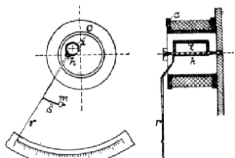
Č. 4658. Voltmetr Hummelův.
