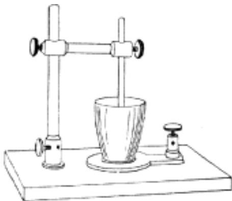
Č. 4655. Voltametr na stříbro.
