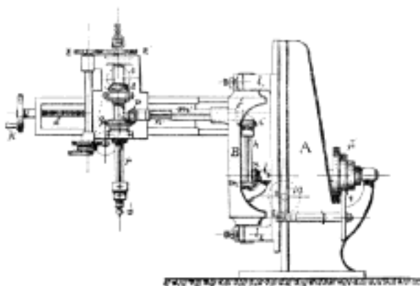
Č. 4678. Radiální stroj vrtací. Č. 4679. Vrtací stroj na dřevu.
