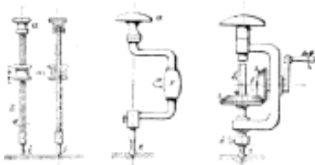
Č. 4673. Svidřík. Č. 4674. Vrtací přístroj prsní. Č. 4675. Vrtací přístroj s ozubeným kolem.
