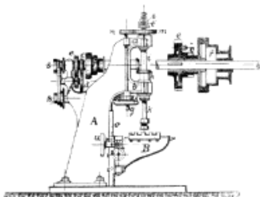
Č. 4677. Vrtací stroj vertikální.
