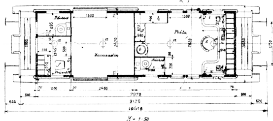
Č. 4708. Dvojosý poštovní vůz s oddělením pro zavazadla a průvodičho.
