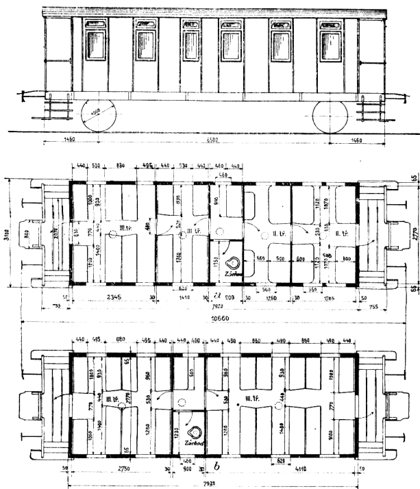
Č. 4709. Dvousový vůz osobní.
