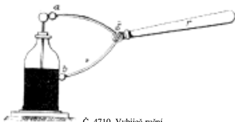
Č. 4710. Vybíječ ruční.
