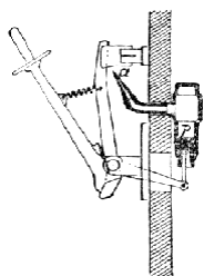
Č. 4720. Vypínač se vzduchovým vypínacem.
