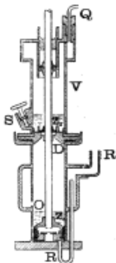
Č. 4740. Vývěva olejová »Guericke«.
