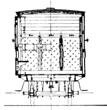
Č. 4704. Vůz pro dopravu koní.
