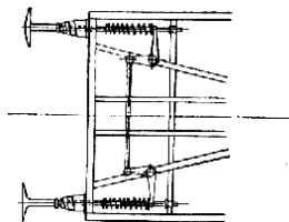
Č. 4699. Nárazník vyrovnávací.
