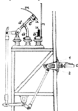
Č. 4721. Vypínač pro vysoké napětí.
