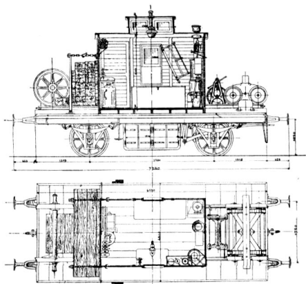
Č. 4705. Výpomocný vůz.
