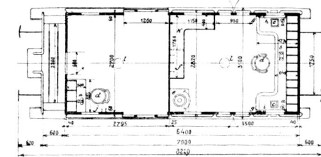
Č. 4707. Dvojosý poštovní vůz s oddělením pro zavazadla.
