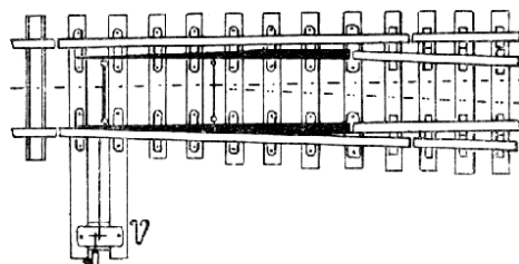
Č. 4713. Výměna hrotitá.
