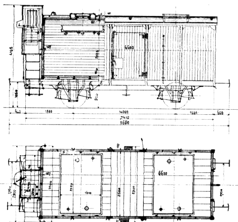
Č. 4703. Vůz pro dopravu nářadí potřebného k udržování a opravě tratí, k opravě porouchaných vozidel apod. a vyobr. č. 4705., t. zv. výpomocný v.,
