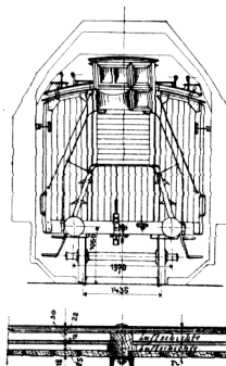
Č. 4703. Vůz pro dopravu nářadí potřebného k udržování a opravě tratí, k opravě porouchaných vozidel apod. a vyobr. č. 4705., t. zv. výpomocný v.,
