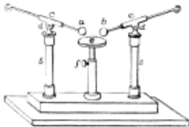
Č. 4711. Henleyův vybíječ.
