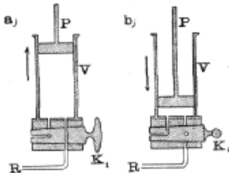
Č. 4739. Vývěva ruční.
