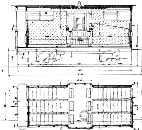
Č. 4704. Vůz pro dopravu koní.
