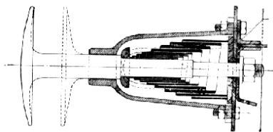
Č. 4698. Nárazník normální.
