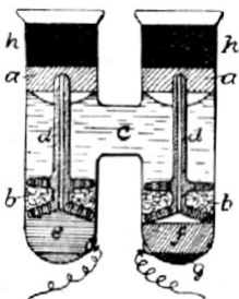
Č. 4748. Westonův článek.
