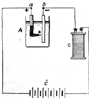
Č. 4746. Wehneltův přerušovač.
