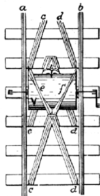
Č. 4749. Wetliho železnice.
