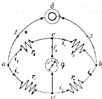
Č. 4750. Princip Wheatstoneova můstku.
