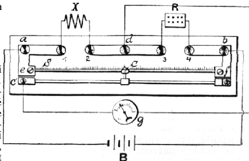
Č. 4751. Wheatstoneův můstek.
