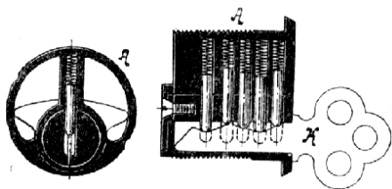
Č. 4779. Yaleův zámek.
