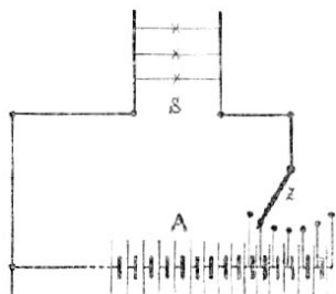
Č. 4784. Jednoduchý zařazovač článkový.
