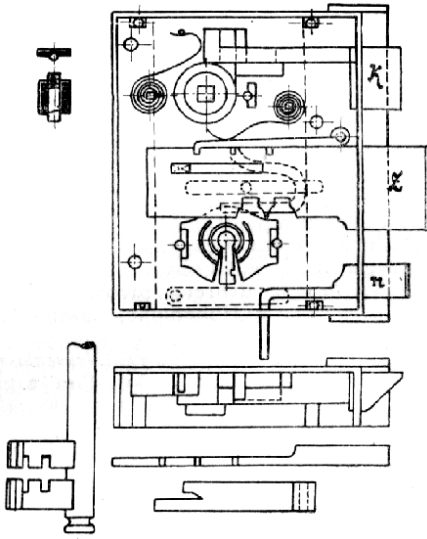
Č. 4776. Závorkový zámek se střelkou.
