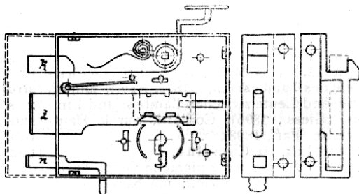
Č. 4775. Francouzský zámek.
