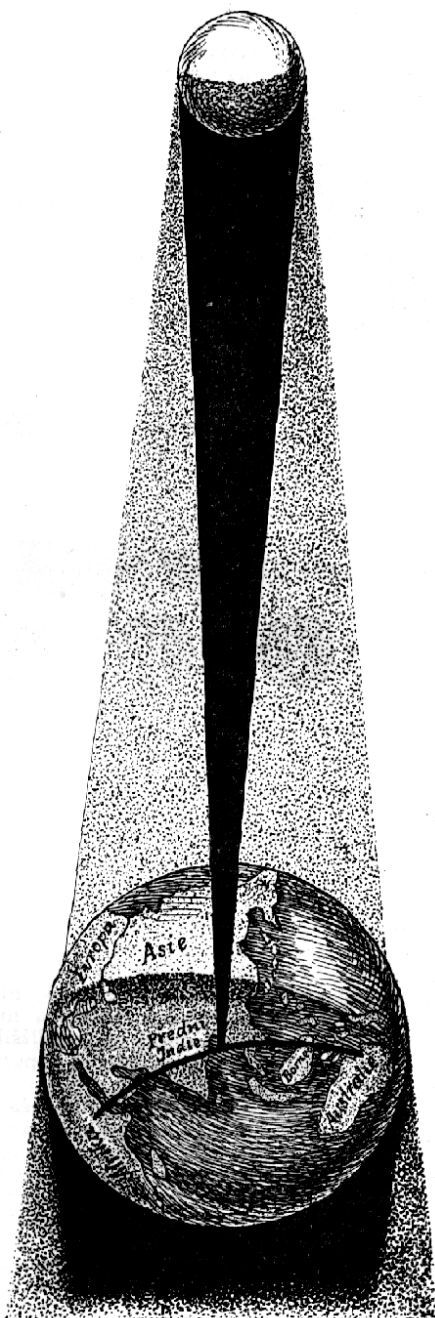
Č. 4793. Průběh úplného zatmění slunce na zemi.
