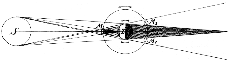
Č. 4791. Zatmění slunce a měsíce.
