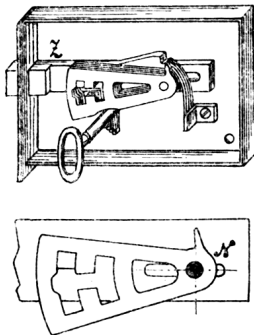
Č. 4777. Zámek Chubbův.
