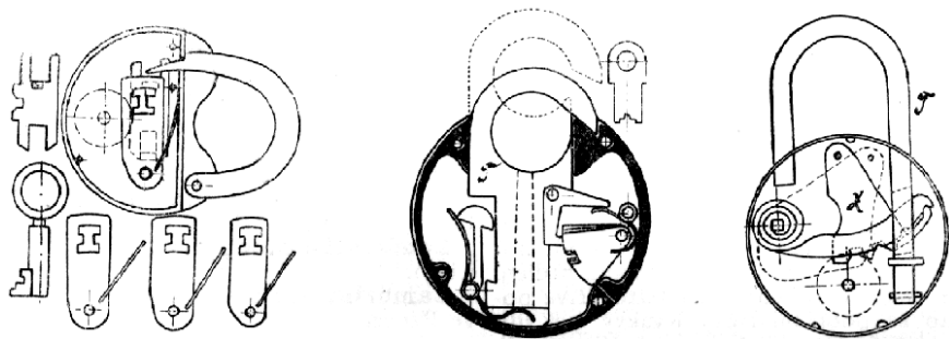
Č. 4774. Visací zámky.
