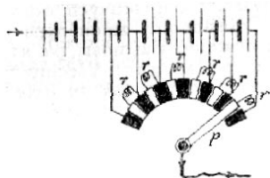
Č. 4786. Starý způsob zařazovače akumulátorového.
