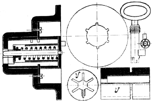
Č. 4778. Bramahův zámek.
