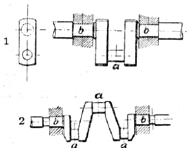
Č. 4773. 1. Jednoduchý hřídel zalomený. - 2. Hřídel trojnásobně zalomený.
