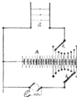
Č. 4785. Dvojitý zařazovač článkový.
