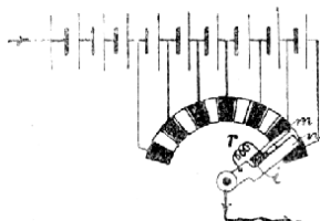
Č. 4787. Zařazovač akumulátorový s jednou odporovou spirálou.
