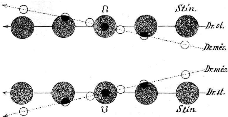
Č. 4792. Polohy měsíce a stínu zemského blízko uzlů.
