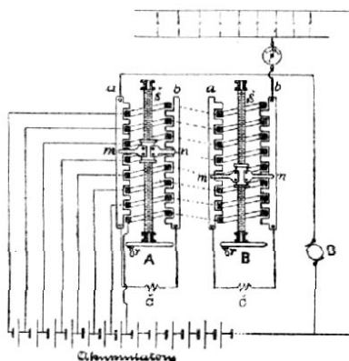
Č. 4789. Posuvný zařazovač dvoujitý.
