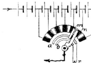
Č. 4788. Novější konstrukce zařazovače s jednou spirálou odporovou.
