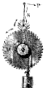
Č. 4798. Ustrojí kolového zdvihadla s jednoduch. převodem.
