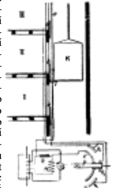
Č. 4808. Automatické zastavování zdviže zapětím odporu v magnetech na krátko.
