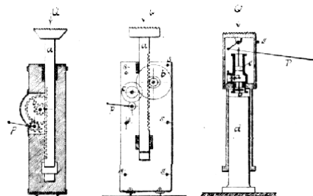
Č. 4804. Vozový č. dřevěný zdvihák.
