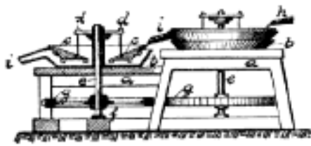
Č. 4814. Amalgamační mlýnek.
