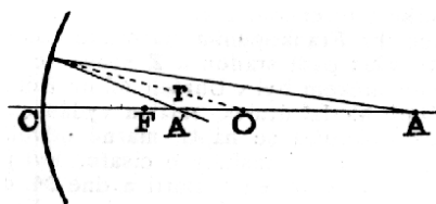
Č. 4830. Duté zrcadlo sférické: Zobrazování bodu.
