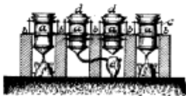
Č. 4819. Plattnerův přístroj.
