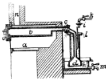
Č. 4816. Retortová pec.
