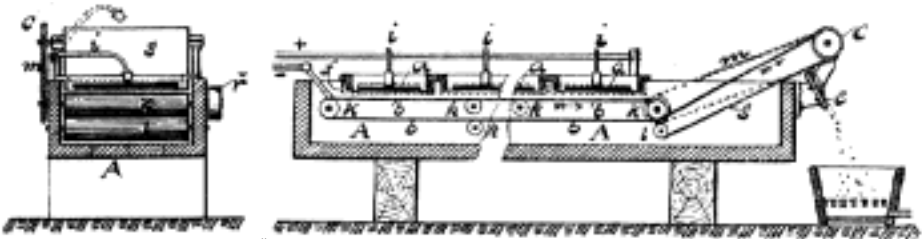
Č. 4822. Elektrolytický přístroj Möbiu v dobývání zlata.
