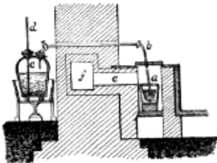
Č. 4823. Millerův přístroj na rafinaci zlata.
