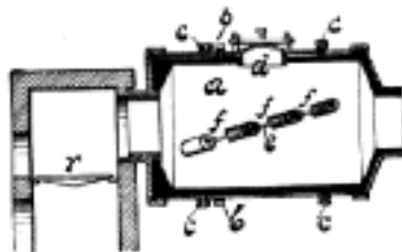
Č. 4818. Brücknerova pec rotační.
