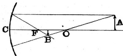
Č. 4831. Duté zrcadlo: Zobrazování předmětu.
