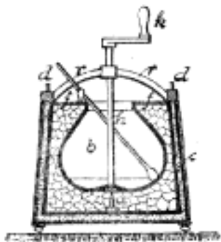
Č. 4825. Fullerův přístroj na zmrzlinu.
