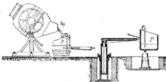
Č. 4870. Plnění a vyprazdňování pánvi při výrobě oceli plávkové.
