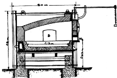
Řez příčný.
