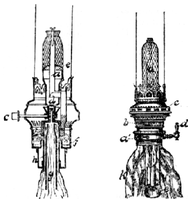
Č. 4856. Lihová lampa žárová »Final«.
