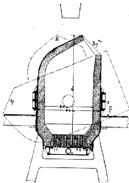
Č. 4868. Konvertor pro bessemerování a thomasování.
