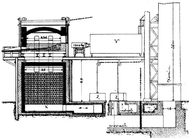
Č. 4874. Příčný řez pecí Siemens-Martinovou.
