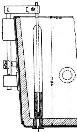
Č. 4869. Řez výtokem slévárenské pánve.
