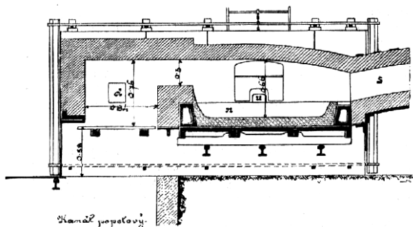
Řez podélný.
