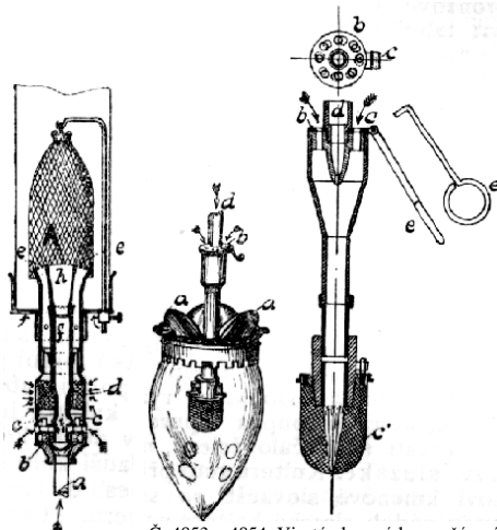
Č. 4852. Žárová lampa »Goliath«.
