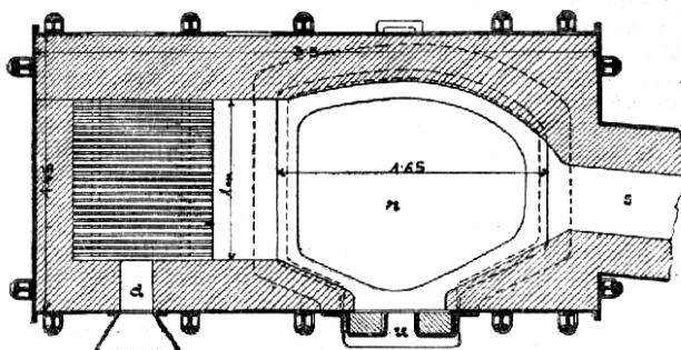
Přídorys.
