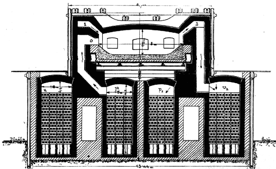
Č. 4873. Podélný řez pecí Siemens-Martinovou a regenerátory.
