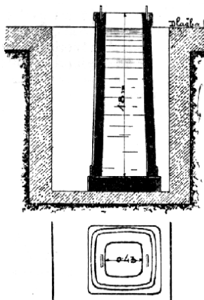
Č. 4871. Pudorys a řez jamou s kokylami.
