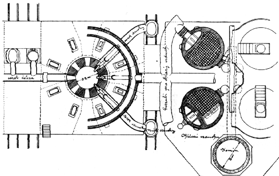
Č. 4865. Moderní vysoká pec s ohřívací větrů.
