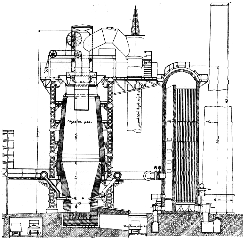
Č. 4864. Moderní vysoká pec s ohřívací větru. (Rez vertikální.)
