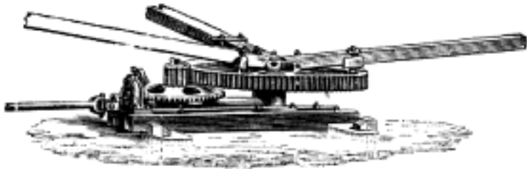
Č. 4879. Žentour ležatý
