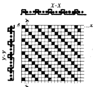
Č. 2186. Kepr outkový čtyřvazný, směr řádků od pravé strany k levé, kde nití outkové kladou se přes 3 nití osnovní na povrch látky a také jen pod 1. nit osnovní na spodní straně látky, tak že jsou 3/4 outku na povrchu. Rez x-x jest veden nití outkovou, y-y nití osnovní.
